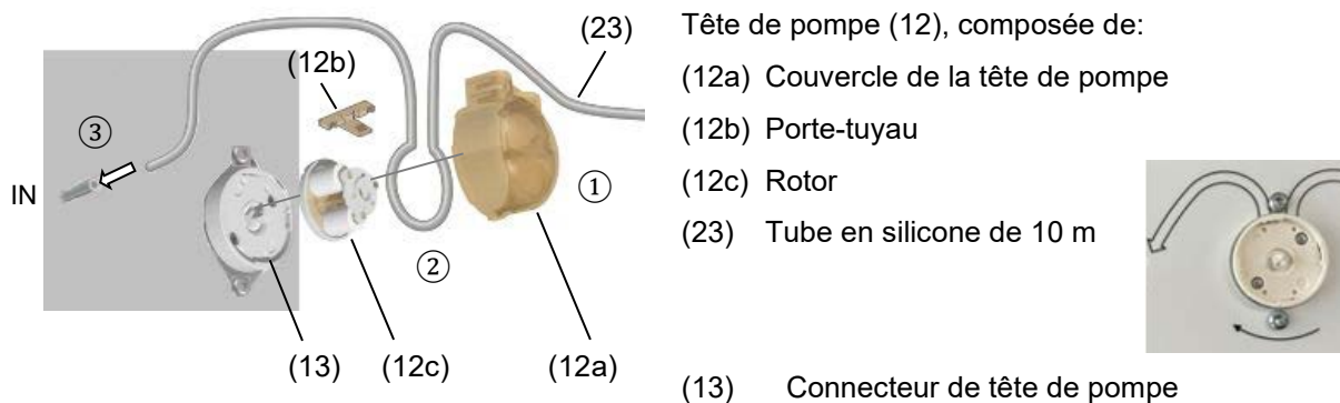
Figure 27: Installation de l'alimentation en eau à la pompe
