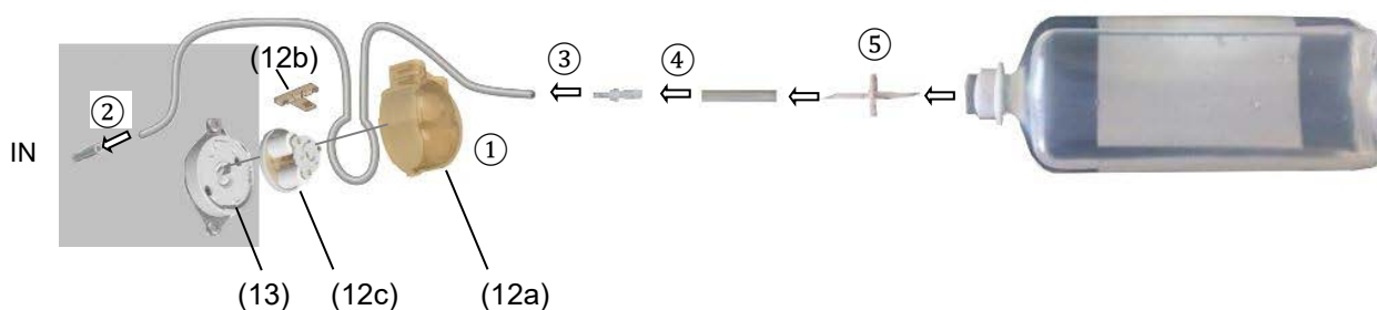
Figure 21: Installation de l'alimentation en eau par bouteille d'eau remplie
