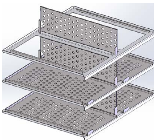
Figure 39 : Support de clayettes, les cloisons de séparation installés (exemple volume 170)
