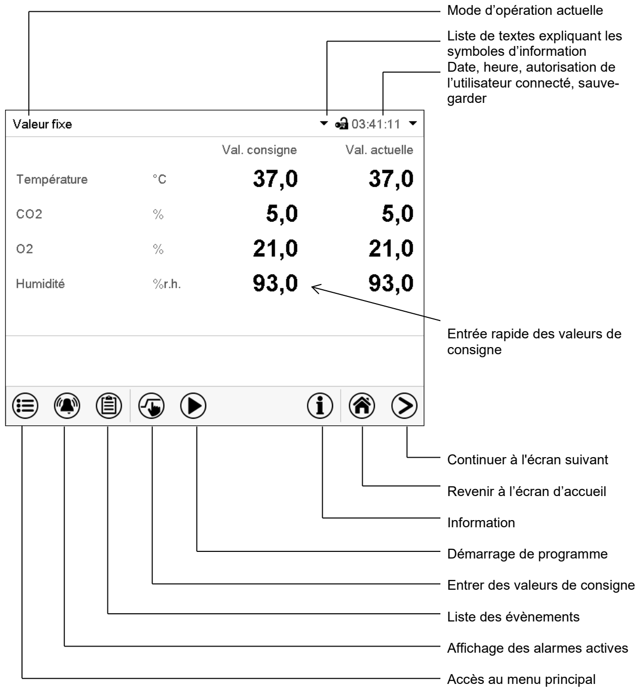
Figure 41: Fonctions d'opération du régulateur MB2 dans l'écran d'accueil (valeurs d'exemple, CBF / CBF-UL avec réglage d'O 2 )
