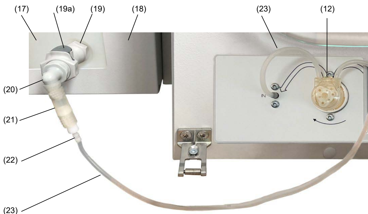
Figure 29: Installation de l'alimentation en eau par la nourriture d'eau fraîche, exemple d'appareil unique
