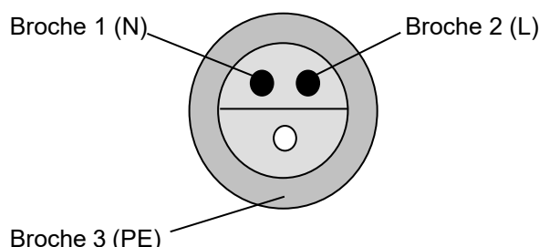
Figure 49: Prise fournie étanche à l'eau (vue avant)
