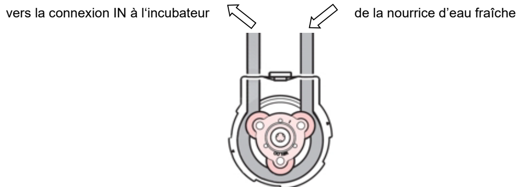
Figure 28: Insertion du tuyau en silicone dans la tête de pompe ②
