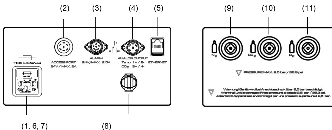
Figure 10: Panneau de connexion CB 170, CBF 170 au dos de l'appareil avec réglage d'O 2 et des options
