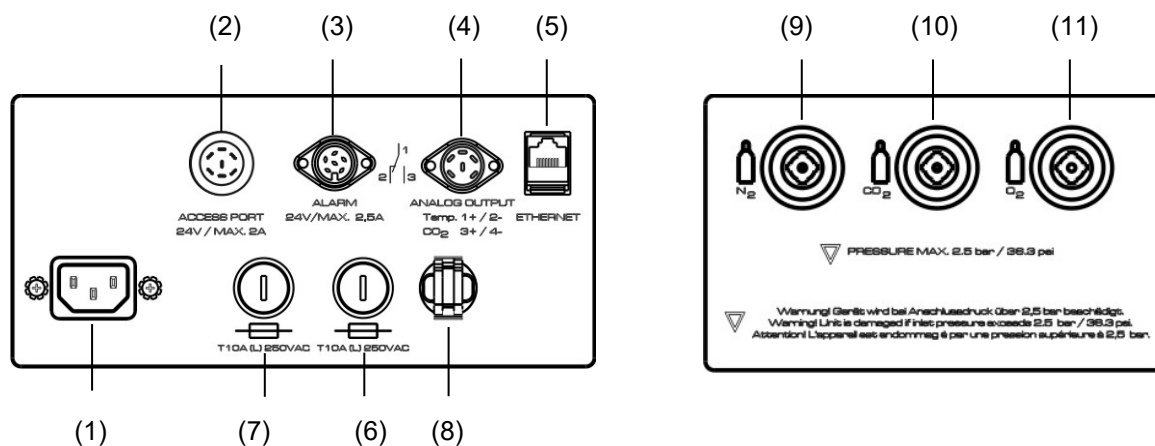
Figure 9: Panneau de connexion CB / CBF au dos de l'appareil avec réglage d'O 2 et des options
