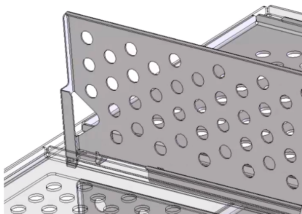
Figure 38 : Cloison de séparation vol. 170 / 260, branché
