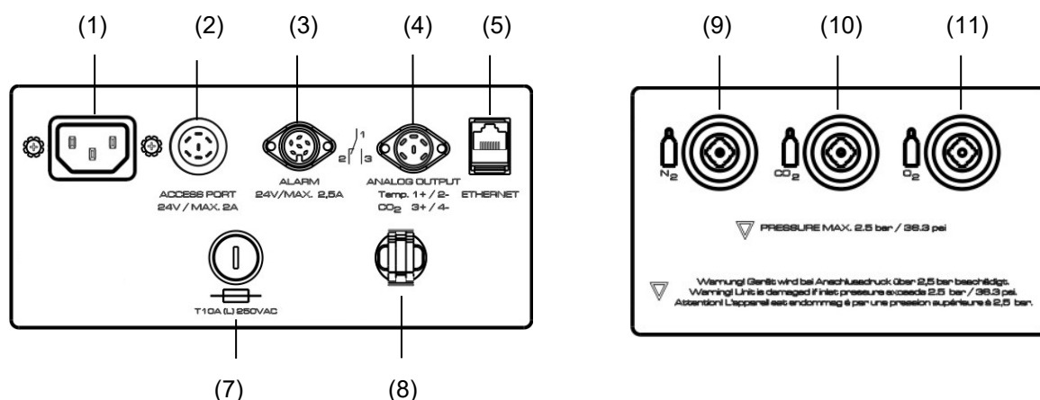
Figure 11: Panneau de connexion CB-UL / CBF-UL au dos de l'appareil avec réglage d'O 2 et des options
