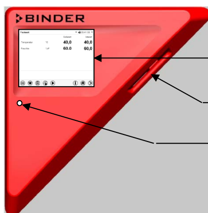
Figure 12: Panneau d'instrumentation triangulaire Régulateur de programmes MB2 et l'interface USB
