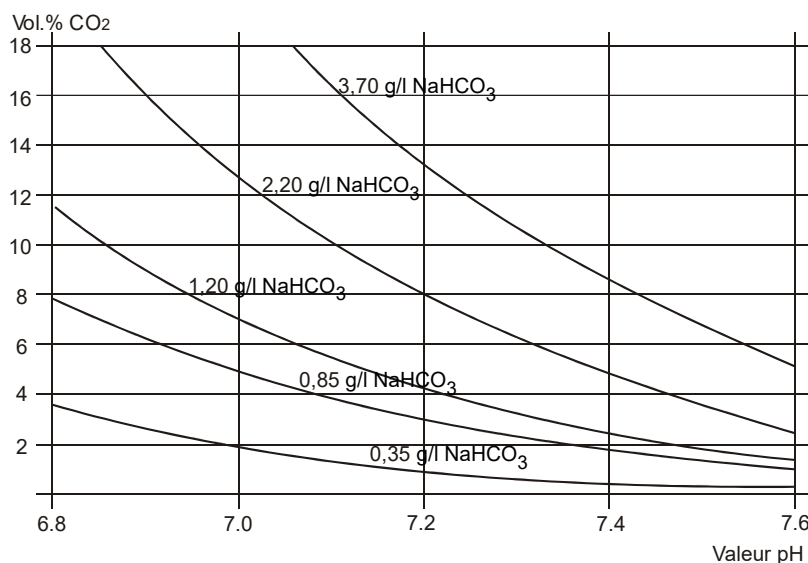
Figure 53: Valeur pH des bouillons courants de culture, tamponnés par \text{NaHCO}_3 en fonction de la concentration en \text{CO}_2
