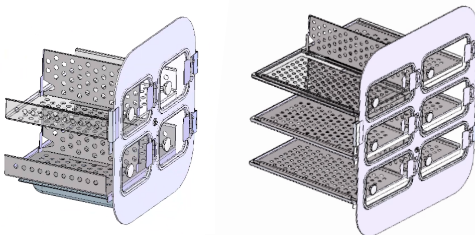
Figure 33 : Porte intérieure divisée avec les clayettes et les cloisons de séparation (exemple pour les appareils vol. 56 et 170)
