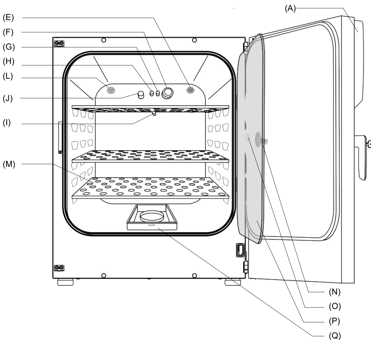
Figure 7: Incubateur CB 170 avec réglage d'O 2 et des options
