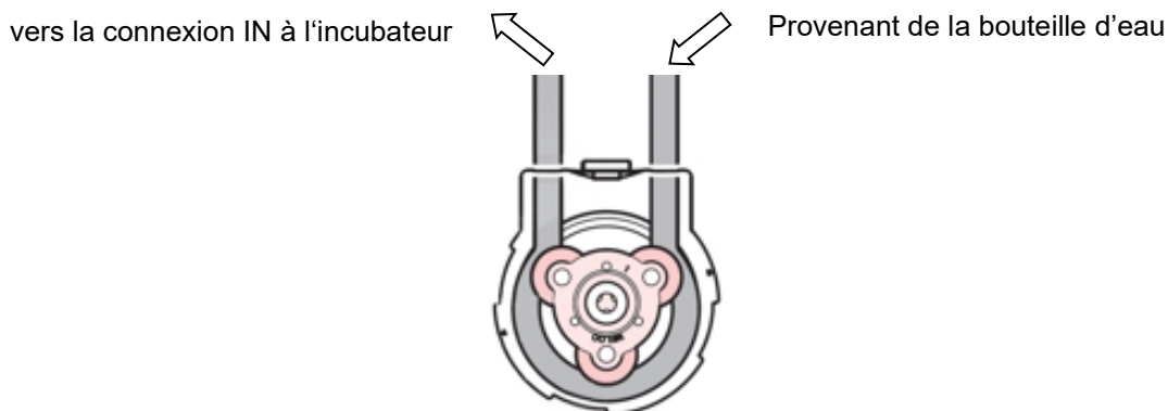
Figure 22: Insertion du tuyau en silicone dans la tête de pompe ②
