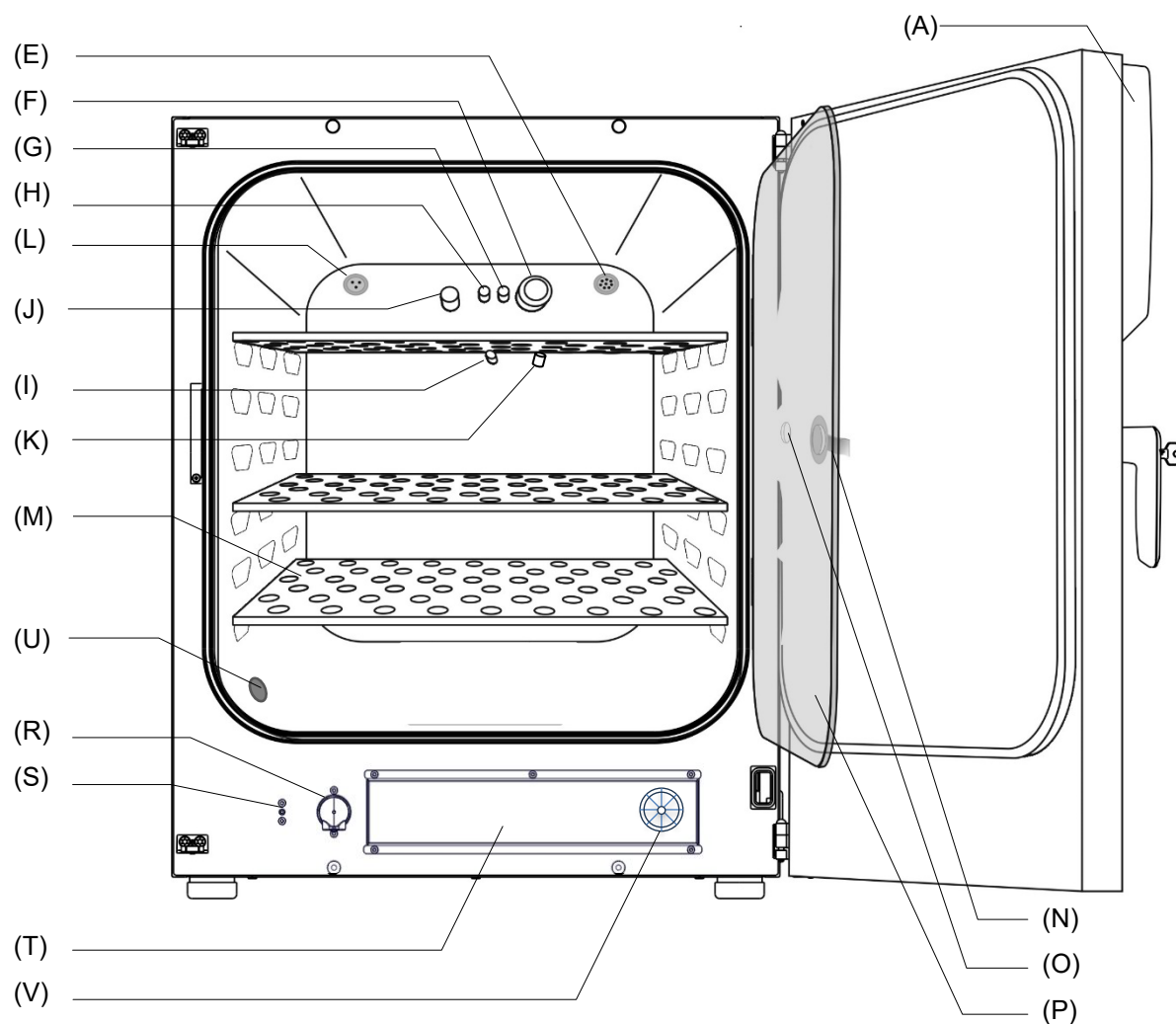
Figure 8: Incubateur CBF 170 avec réglage d'O 2 et des options
