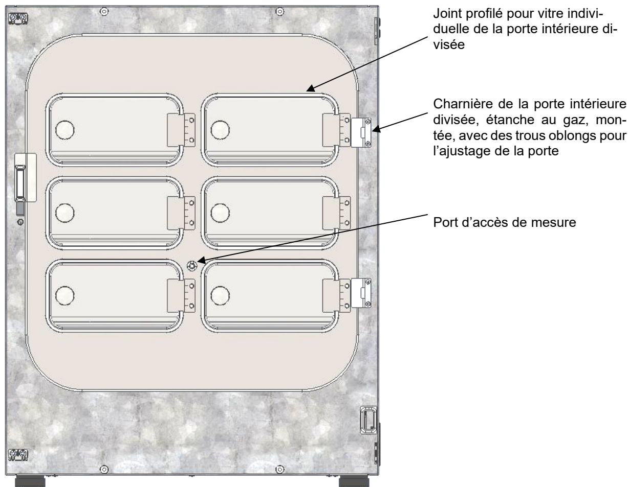
Figure 32: Porte intérieure divisée (exemple : CB 170)
