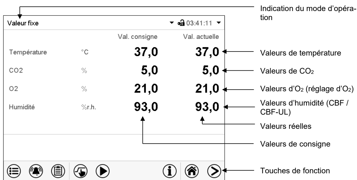
Figure 40: Écran d'accueil du régulateur programmable MB2 (valeurs d'exemple, CBF / CBF-UL avec réglage d'O 2 active)
