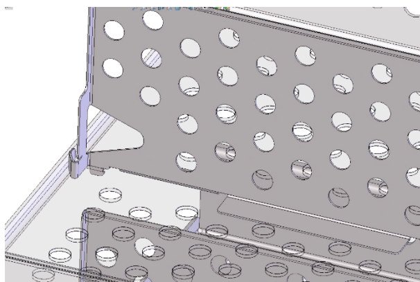
Figure 37 : Cloison de séparation vol. 56, branché
