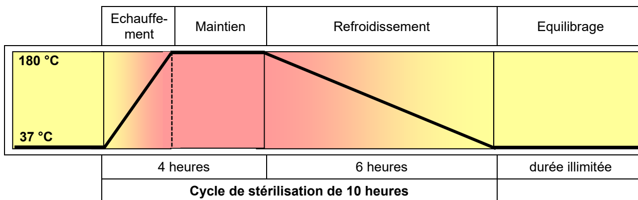
Figure 54: Cours de la valeur de consigne pendant le cycle de stérilisation
