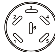
Figure 44: Affectation des pins de la douille DIN (3) au dos de l'appareil
