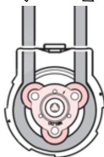
Figure 25: Insertion du tuyau en silicone dans la tête de pompe ①
