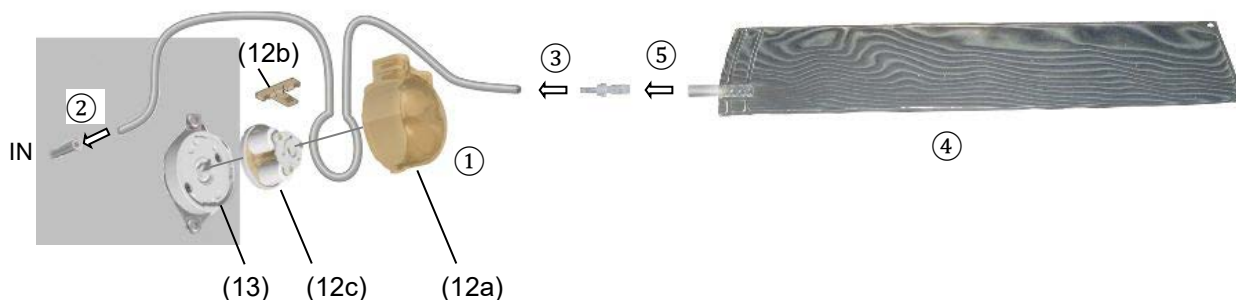
Figure 24: Installation de l'alimentation en eau par sac d'eau douce
