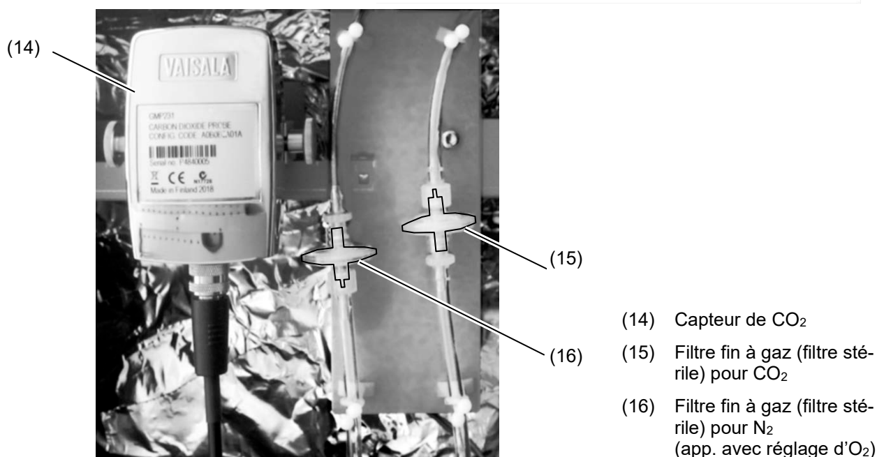
Figure 56: Position du capteur de CO 2 et des filtres fins à gaz derrière le couvercle
