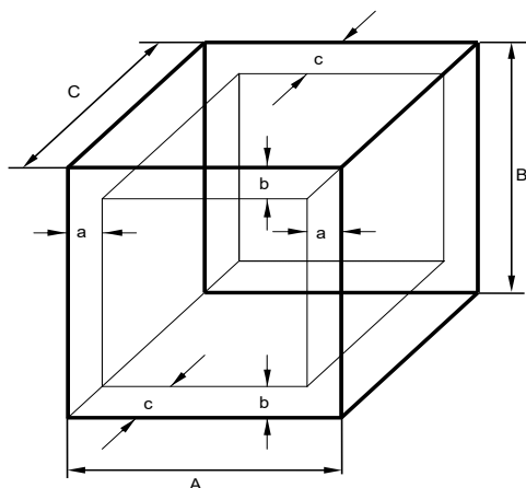
Figure 57: Détermination du volume utile
