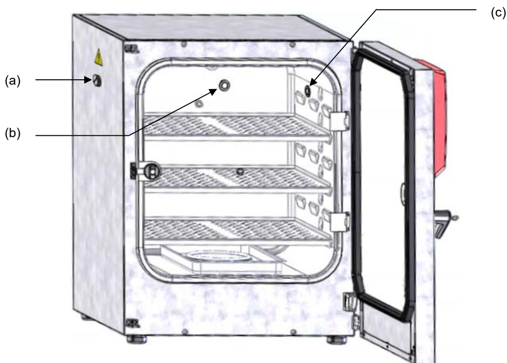
Figure 45: Positions des ports d'accès en silicone optionnels à gauche (a), à l'arrière (b) et à droite (c)
