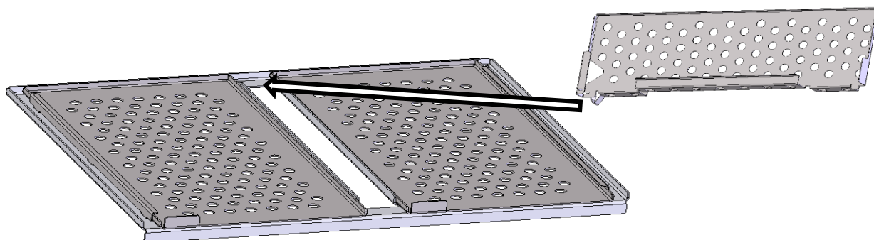
Figure 36 : Insertion de la cloison de séparation
