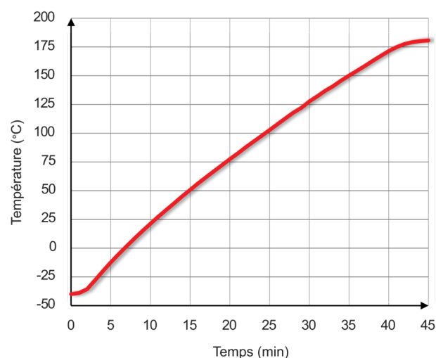
Courbe de chauffage: MKF 720 CO 2
