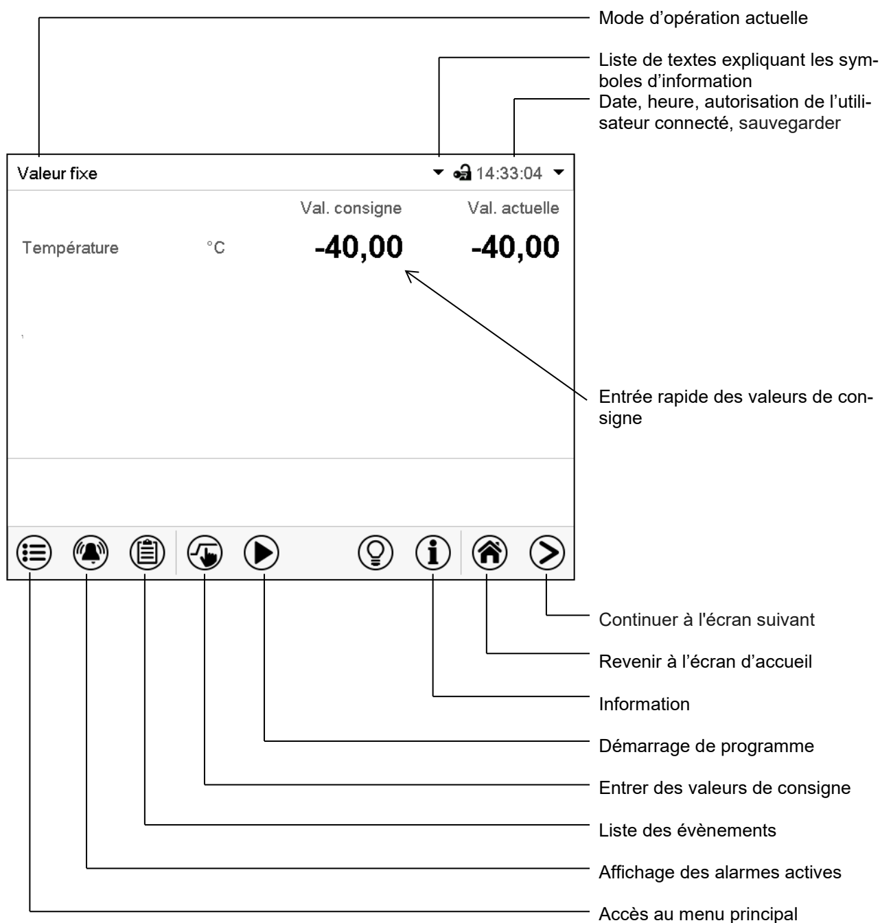
Figure 13: Fonctions d'opération du régulateur MB2 dans l'écran d'accueil (valeurs d'exemple)
