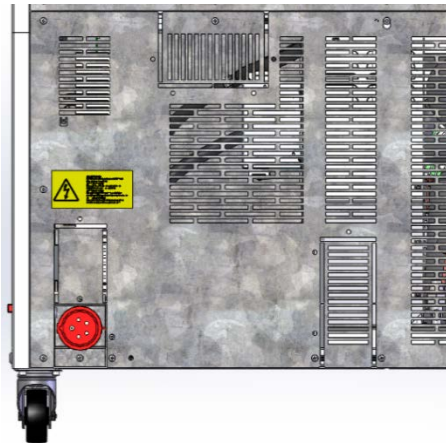
Figure 2: Position du signes de sécurité concernant des disjoncteurs de courant résiduel sur le dos de l'appareil
