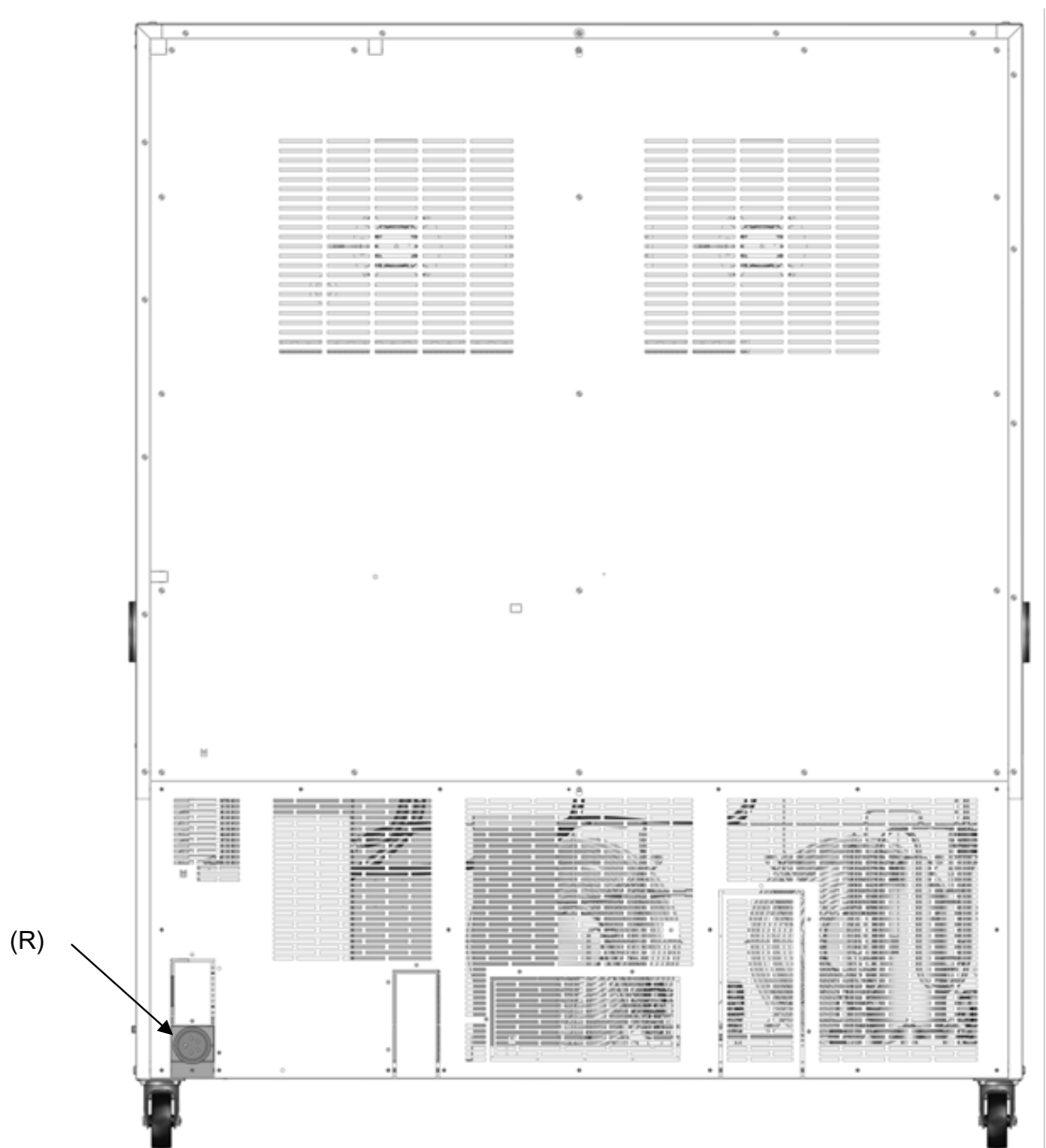
Figure 10: Vue d'arrière (exemple : MK 720)
