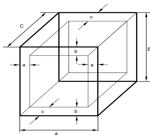
Figure 16: Détermination du volume utile
