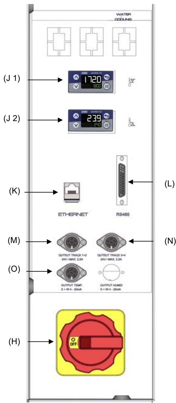
Figure 9: Tableau d'instruments latéral au côté droit du compresseur frigorifique avec des options
