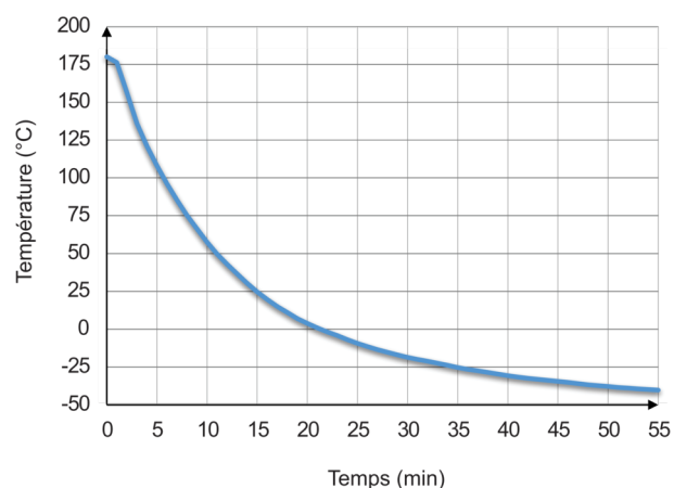
Courbe de refroidissement: MK 240 CO 2
