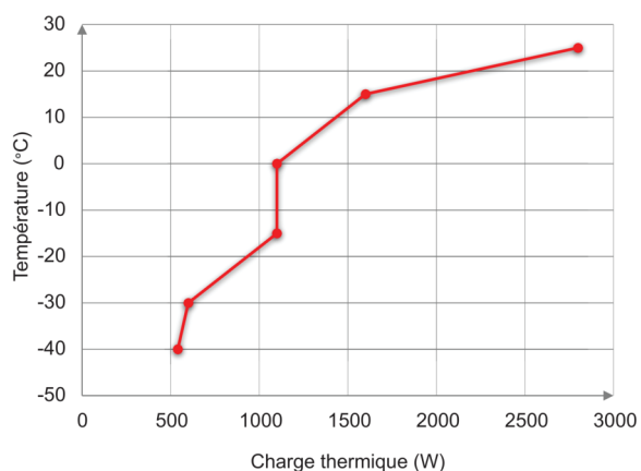
Diagramme de la compensation thermique
